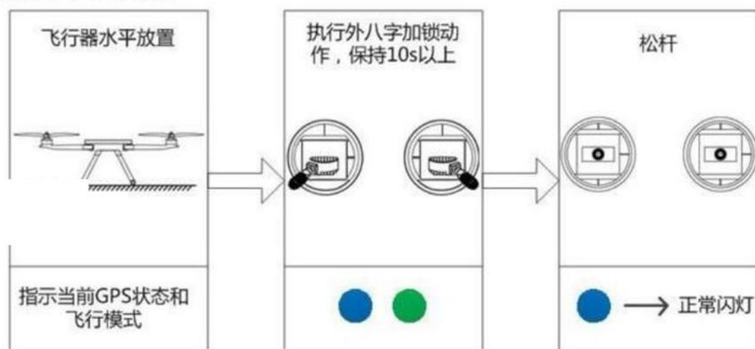
图 2-16 水平校准
