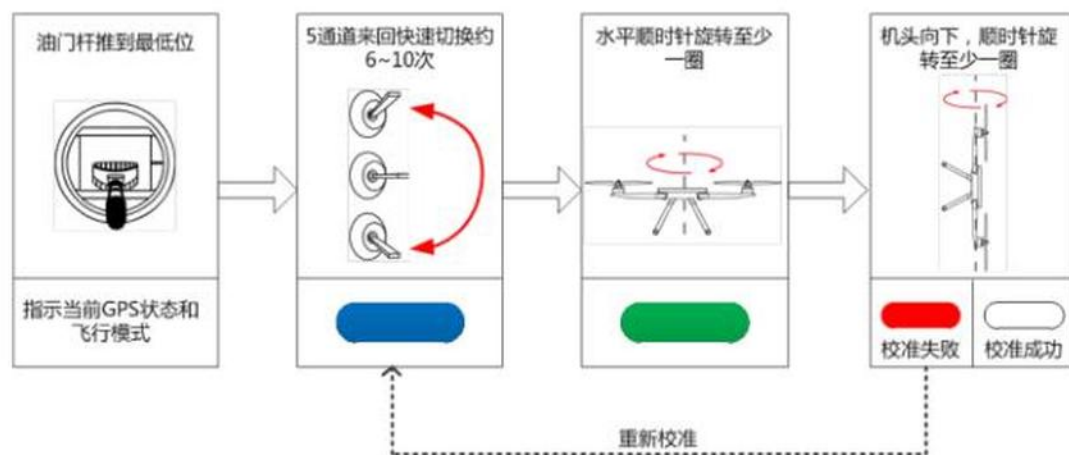
图 2-15 指南针校准
